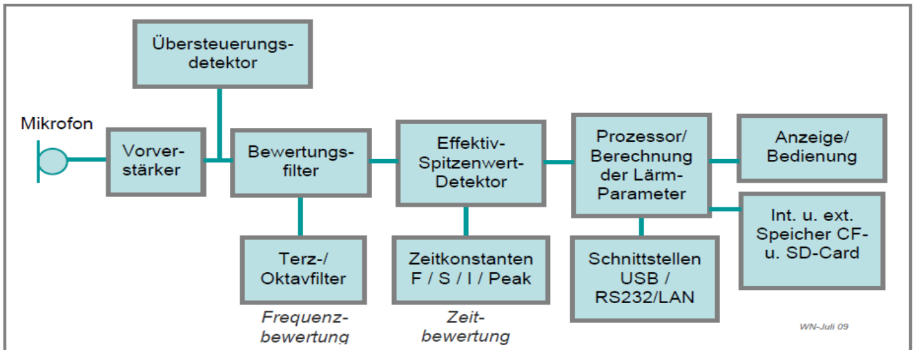
Abb.1 Blockschaltbild eines modernen Schallpegelmessers
