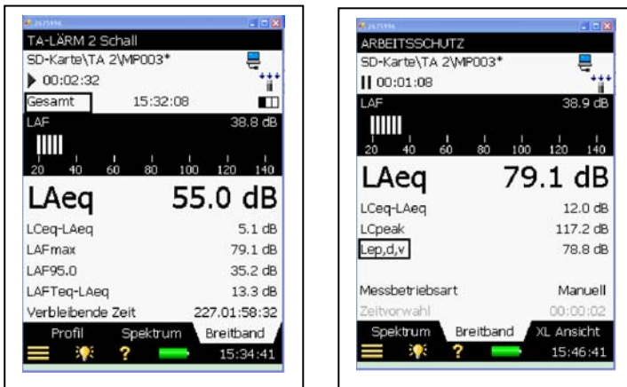
Abb.7 Typische Messparameteranzeige, links typisch für Messungen im Umweltschutz, rechts für Arbeitsschutz
